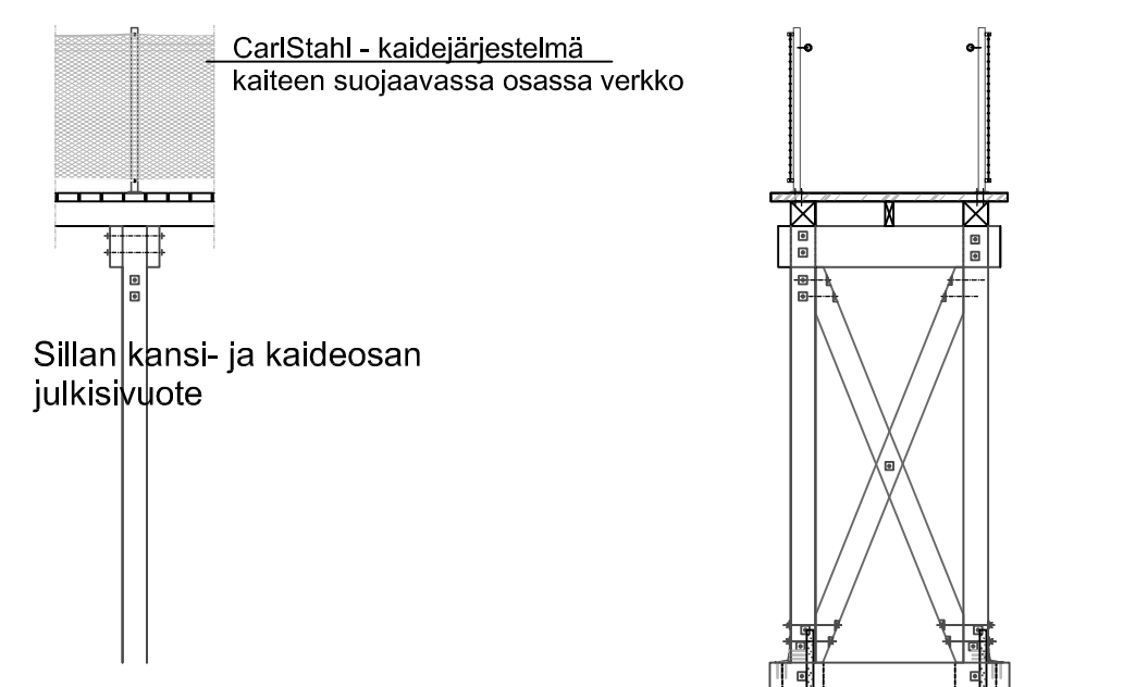
Leikkaus A - A 1:50
